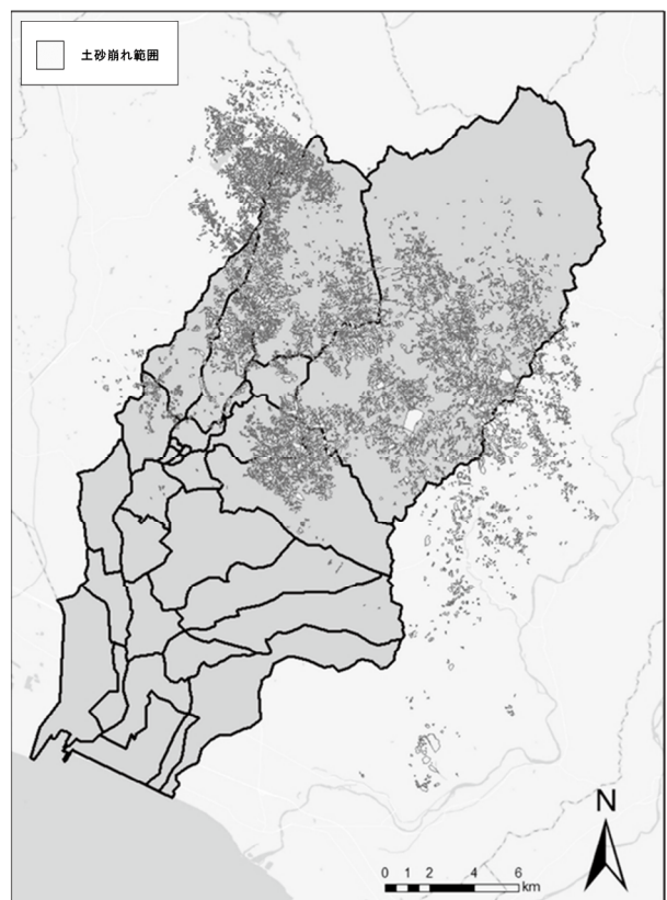
図3 北海道胆振東部地震による土砂崩れの範囲
